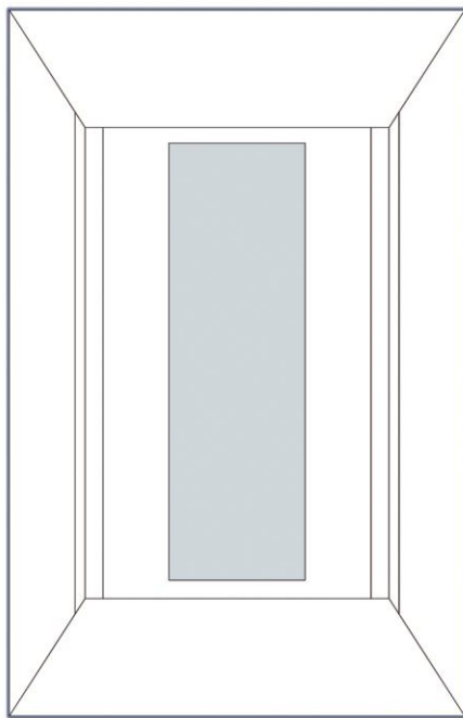
SAP34 | Parete 3/4 Larghezza parziale Altezza totale
